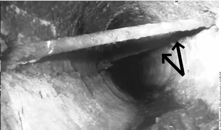
Wnętrze kanału, w którym znajdują się dwa niezainwentaryzowane rurociągi.
